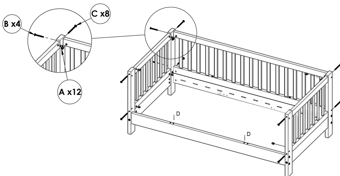
C - M6 x 100 - 8 pcs
