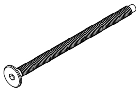
C - M6 x 100 - 8 pcs
